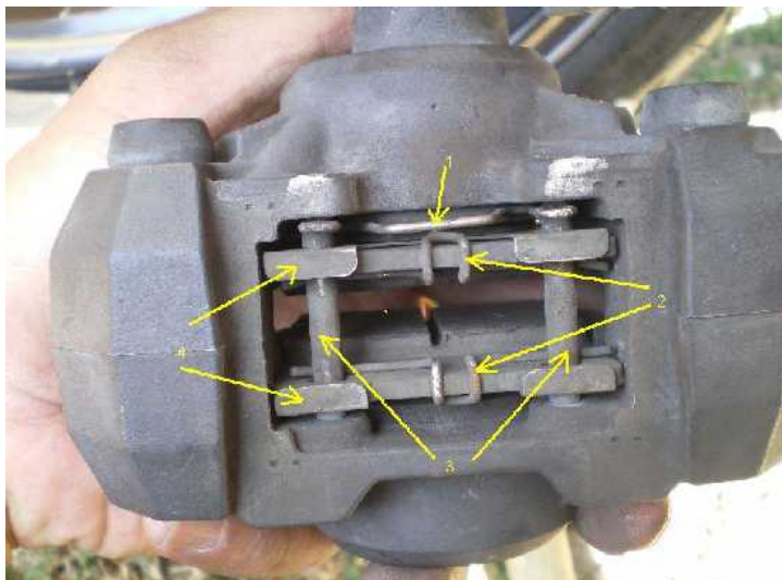
...ecco cosa troviamo sotto il coperchio... dall'alto in senso orario: la copiglia di sicurezza (1), le molle (2), i perni (3), le piastrine delle pastiglie (4)
